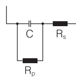
Ersatzschaltung
