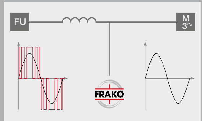
Filter zur Glättung des PWM Signals
