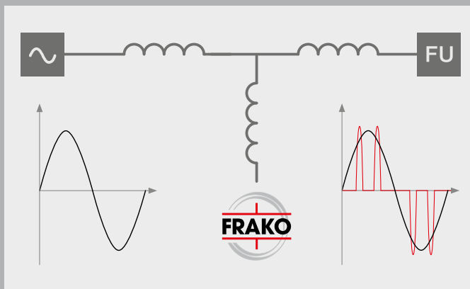
Filter zur Reduzierung der Netzurückwirkungen
